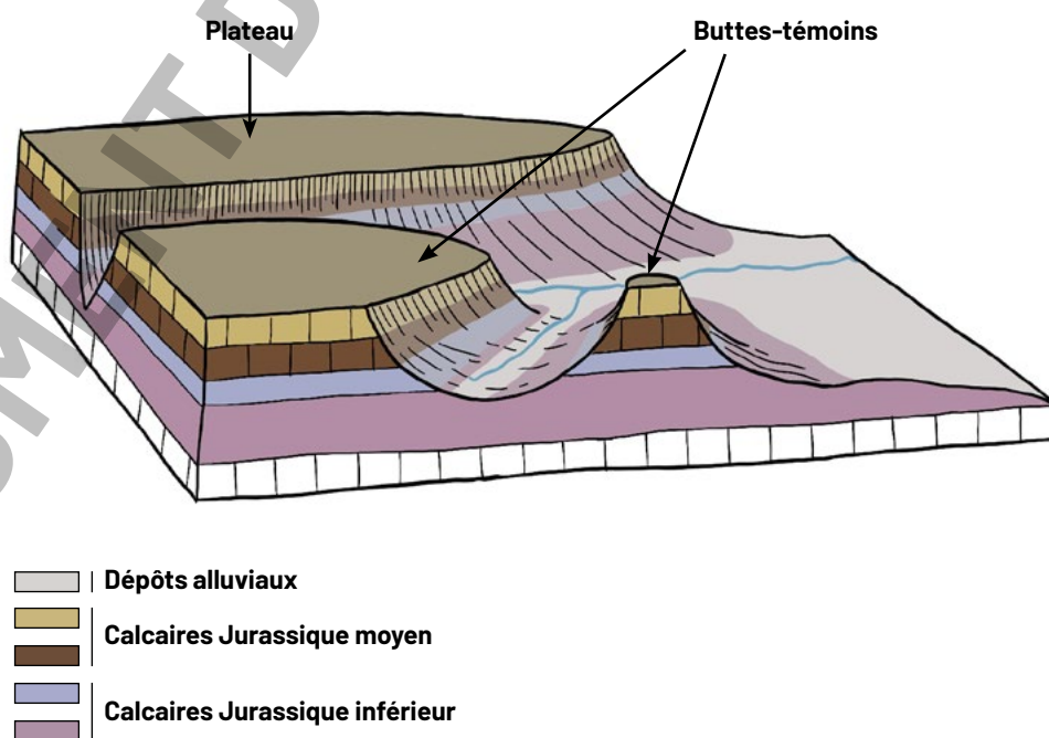
Bloc schématisé de l'organisation géologique du Montbardois (le pendage des couches géologiques n'est pas ici reconstitué avec fidélité).
