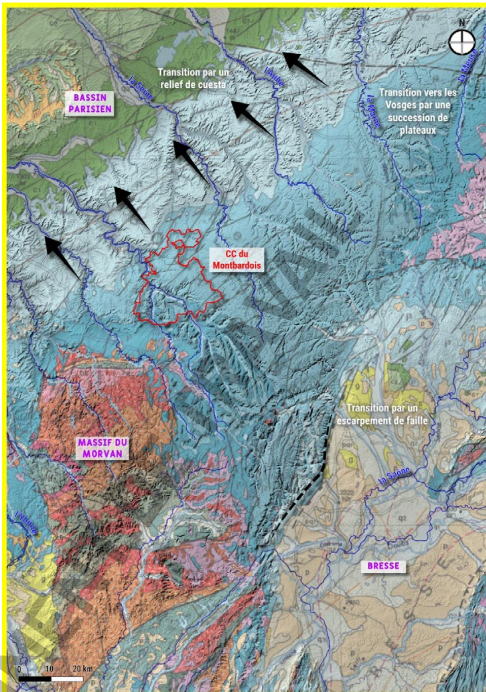
Carte du contexte géomorphologique de la CC Montbardois.
