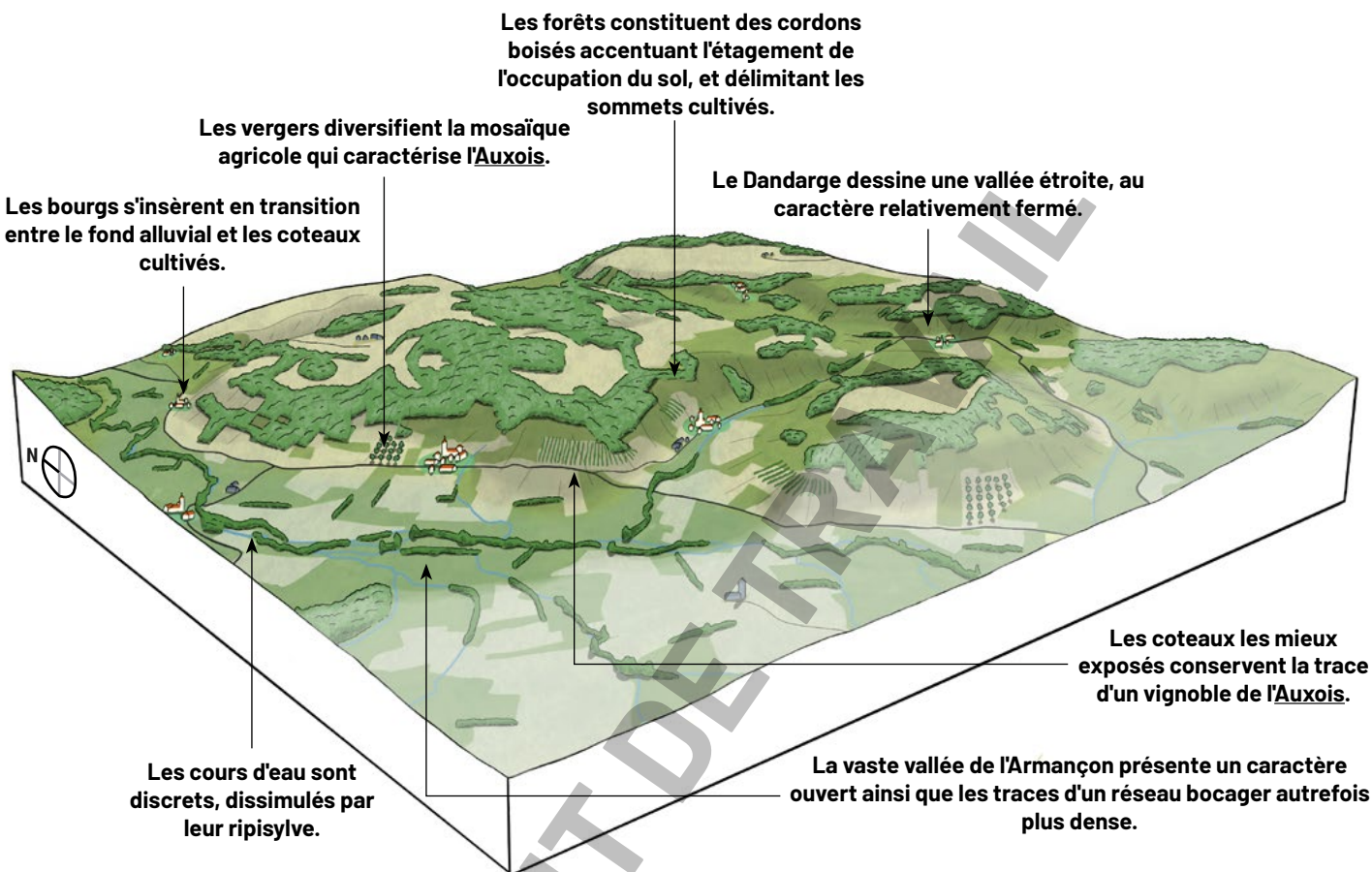
Bloc diagramme de l'unité paysagère de l'Auxois.
