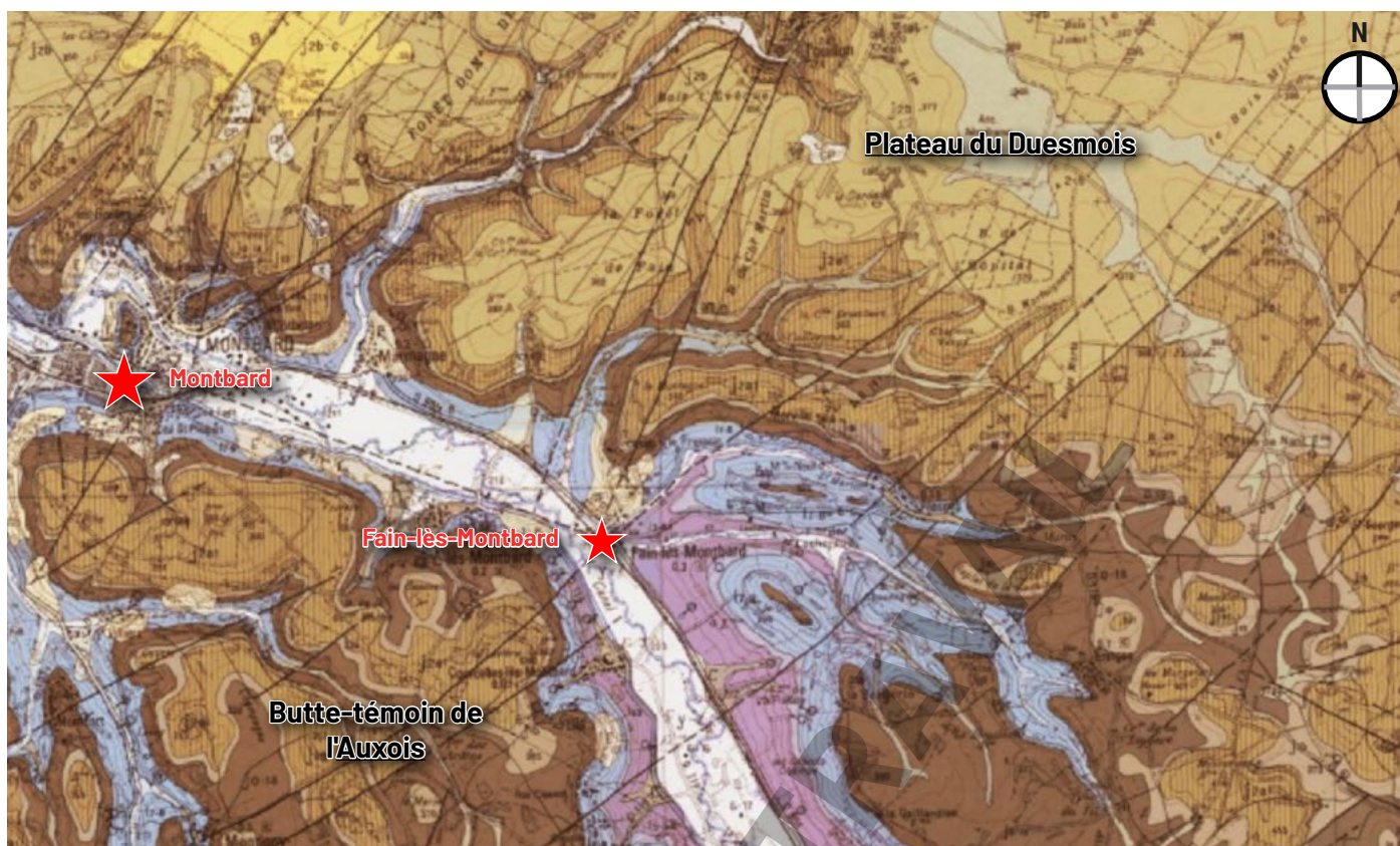
Extrait de la carte géologique au 50 000 ème autour de la vallée de la Brenne, au niveau de Fain-lès-Montbard (source : BRGM, IGN).
