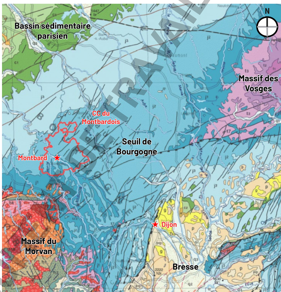
Extrait de la carte géologique au 100 000 ème , au niveau du seuil de Bourgogne (source : BRGM, IGN).
