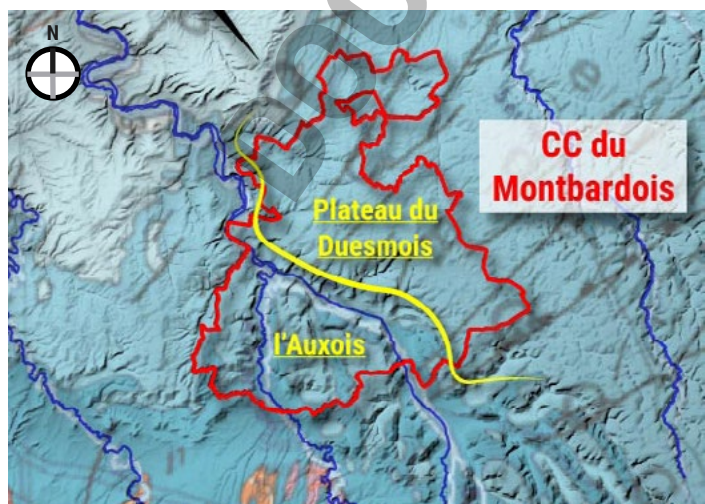
Zoom sur le contexte géomorphologique du Montbardois.
